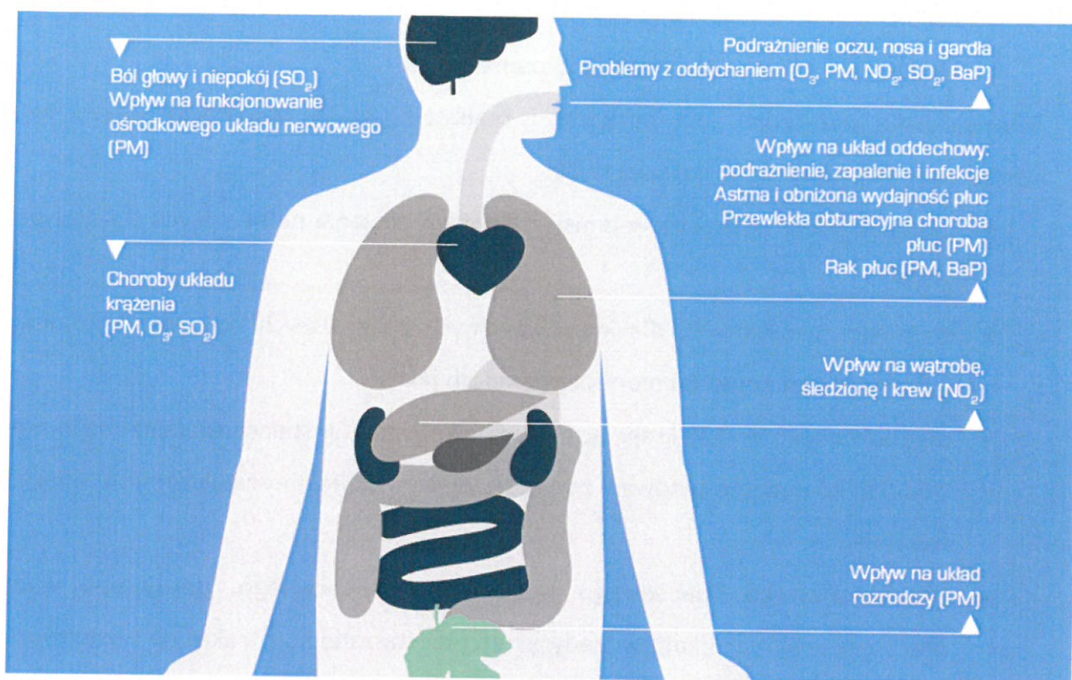
Rys. 3. Oddziaływanie zanieczyszczeń na organizm człowieka.
