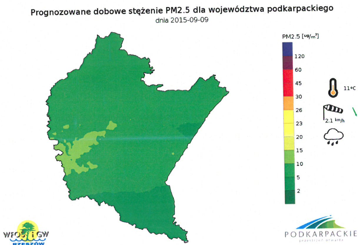
Rys. 7. Prognozowane dobowe stężenie PM2,5.
