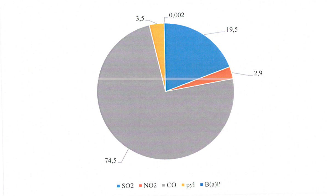
Rys. 12. Struktura emisji zanieczyszczeń.
