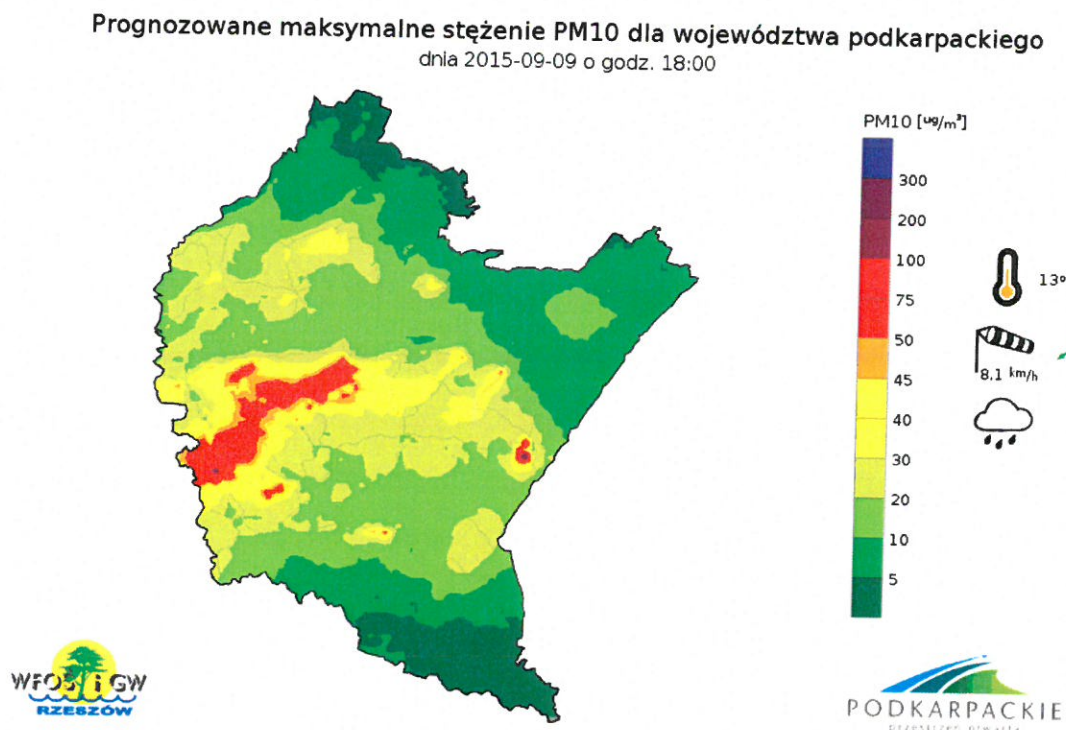
Rys. 6. Prognozowane maksymalne stężenie PM10.
