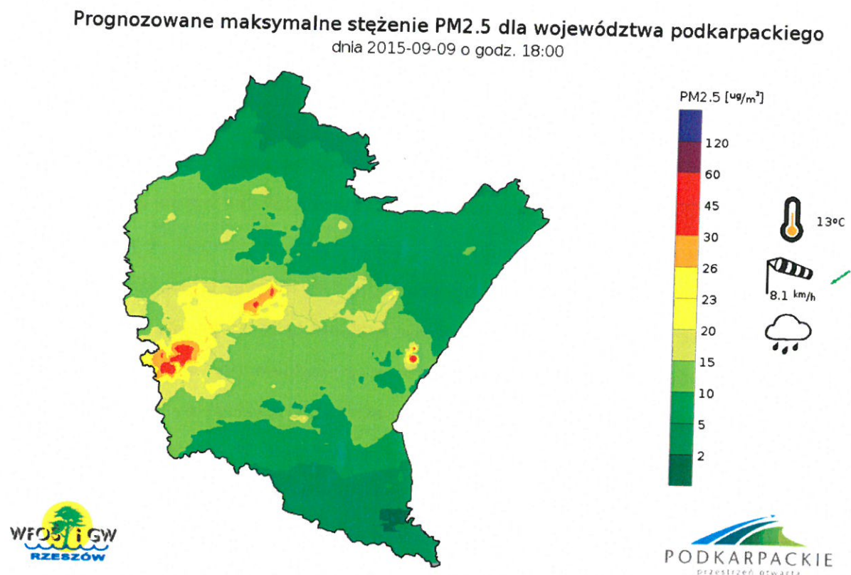
Rys. 8. Prognozowane maksymalne stężenie PM 2,5 .
