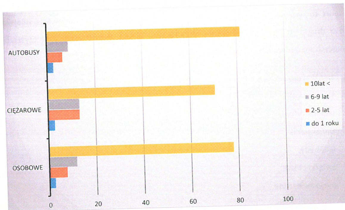
Rys. 2. Wiek pojazdów w Polsce (GUS 2014).
