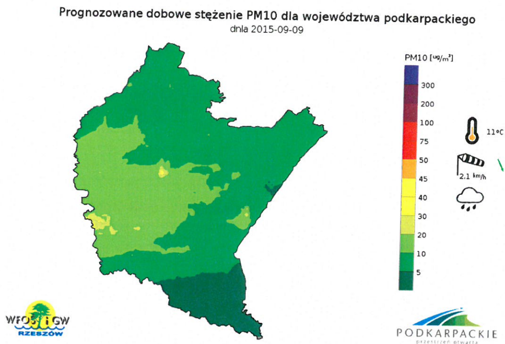
Rys. 5. Prognozowane dobowe stężenie PM10.
